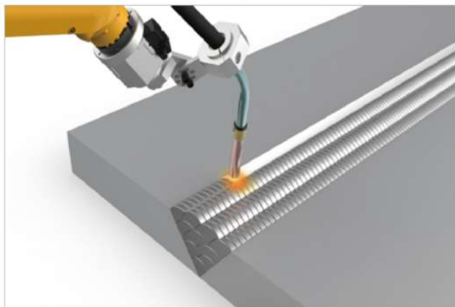
Многослойная многоканальная сварка
